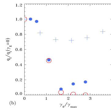
GS2の計算結果(赤丸) [Roach, PPCF(2009)]
