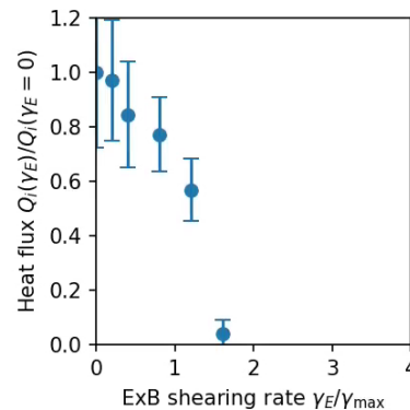
ExBフローシアによる 乱流の安定化 (gkvp_f0.62)
